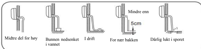
Innendørsenhet
